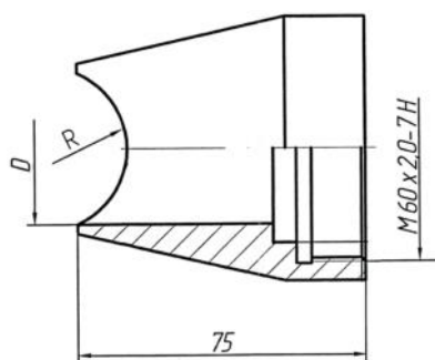
Рис. 13.6 Ниппель переходной для РВД-50 на коллектор
