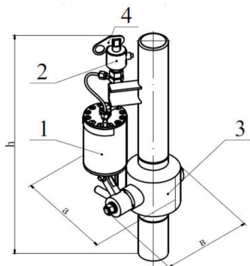
Распределительное устройство (РУА-65-14,7-П-О-24-0К-0-О)
